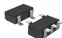
BU4809G-TR Rohm Semiconductor IC VOLT DETECTOR 0.9V SSOP5
